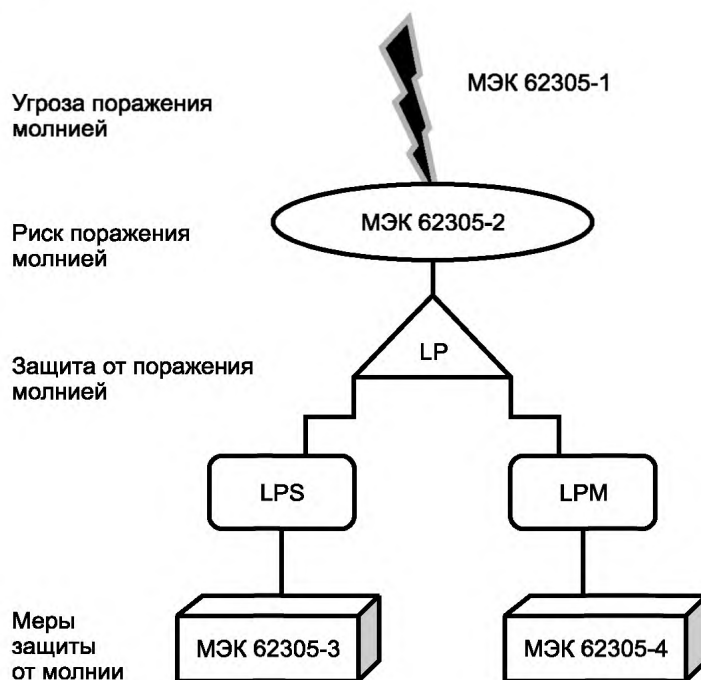
Рисунок 1 — Взаимосвязь стандартов серии МЭК 62305 по применению мер защиты от молнии
