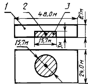
1 — помещение; 2 — аппарат; 3 — взрывоопасная зона
